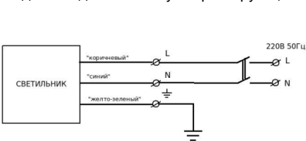
Рисунок 1. Электрическая схема подключения.
