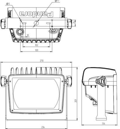
Рисунок 2. Габаритный чертеж
