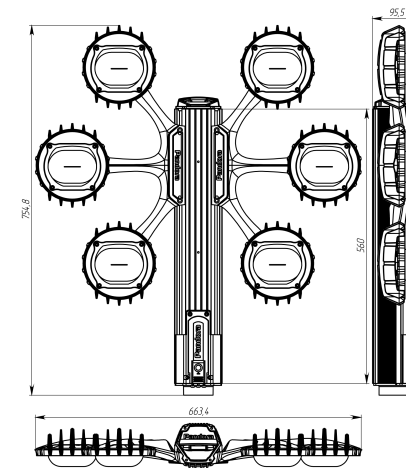
Рисунок 3. Габаритный чертеж
