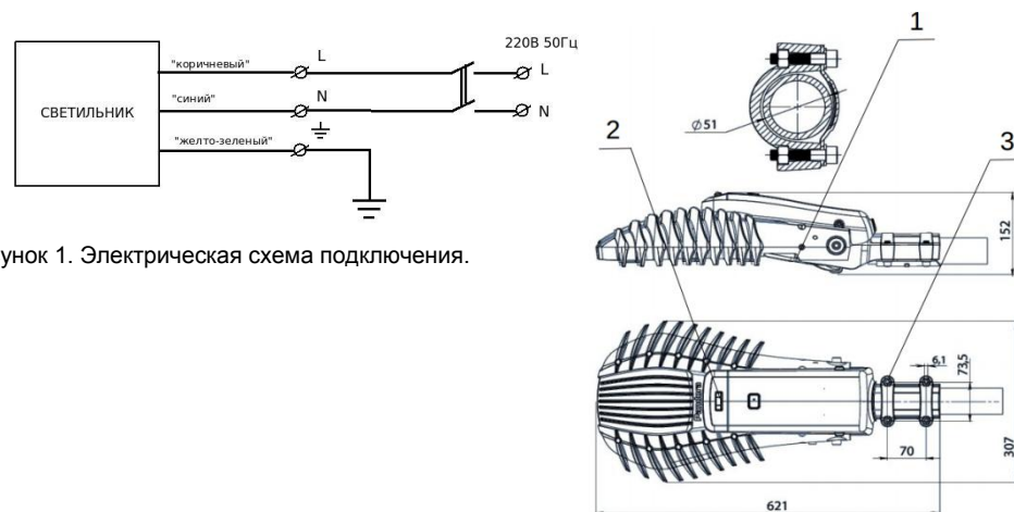
Рисунок 2. Схема установки светильника на кронштейн.
