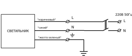
Рисунок 1. Электрическая схема подключения.
