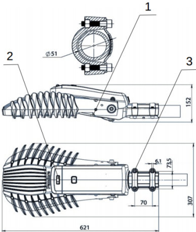
Рисунок 2. Схема установки светильника на кронштейн.
