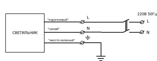
Рисунок 1. Электрическая схема подключения.
