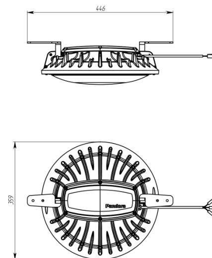
Рисунок 1. Габаритный чертеж.
