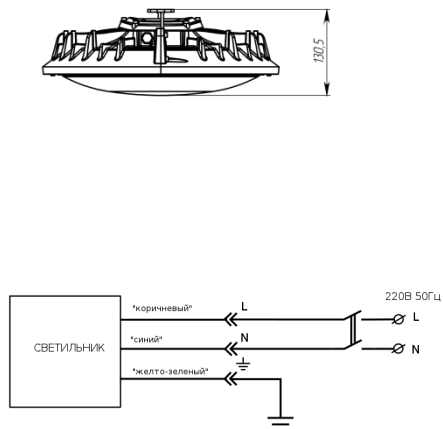
Рисунок 2. Электрическая схема подключения
